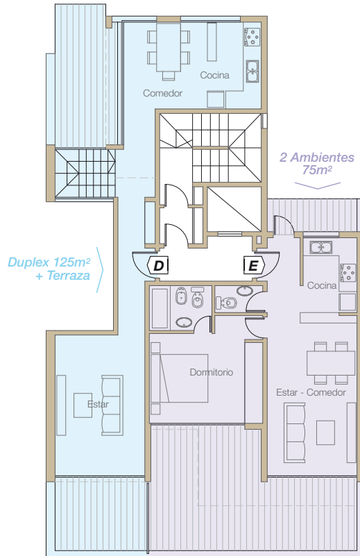
PLANTA 6º
