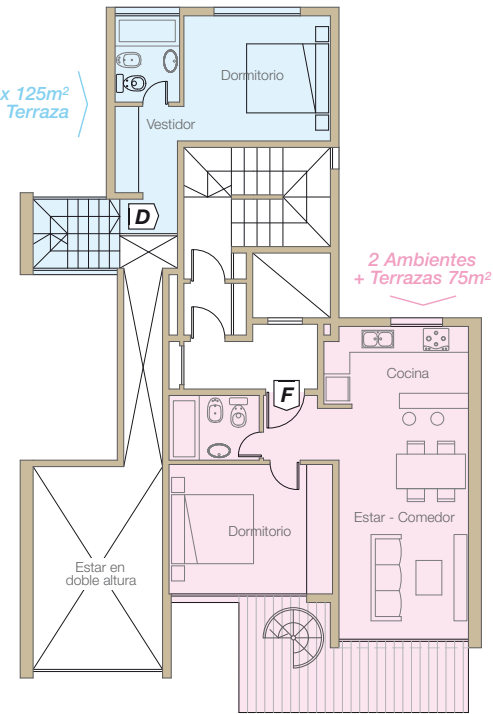
PLANTA 7º
